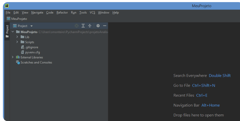
IDE PYCharm.
