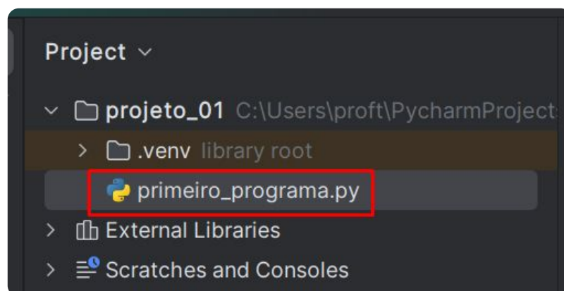
Primeiro_programa.py.
